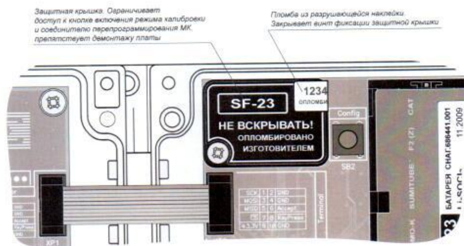
Рисунок 2 - Схема пломбирования защитной крышки корректоров объема газа «Суперфлюу 23»
